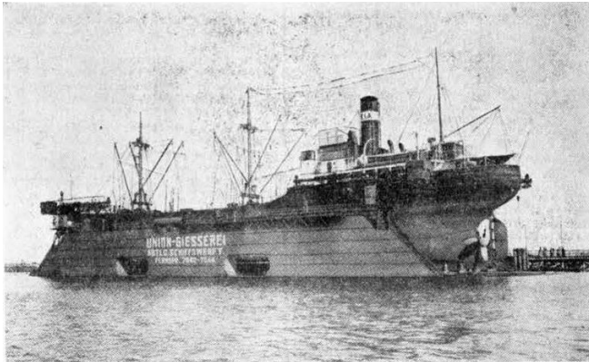
Schwimmdock von 2800 Tonnen Tragfähigkeit, 90 m Länge, 20 m breit Aufn.: Archiv
